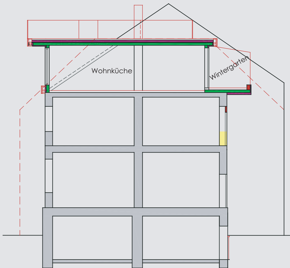
SCHNITT A-A
