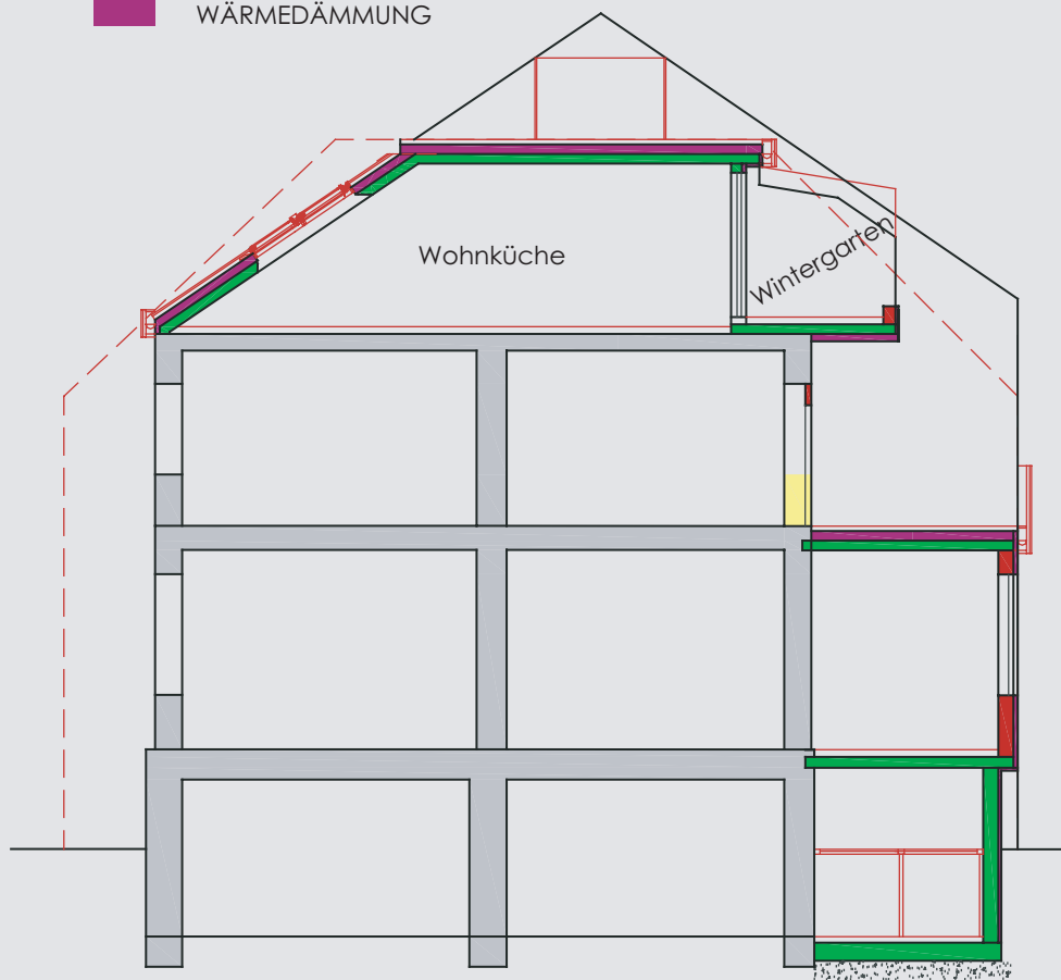
SCHNITT B
